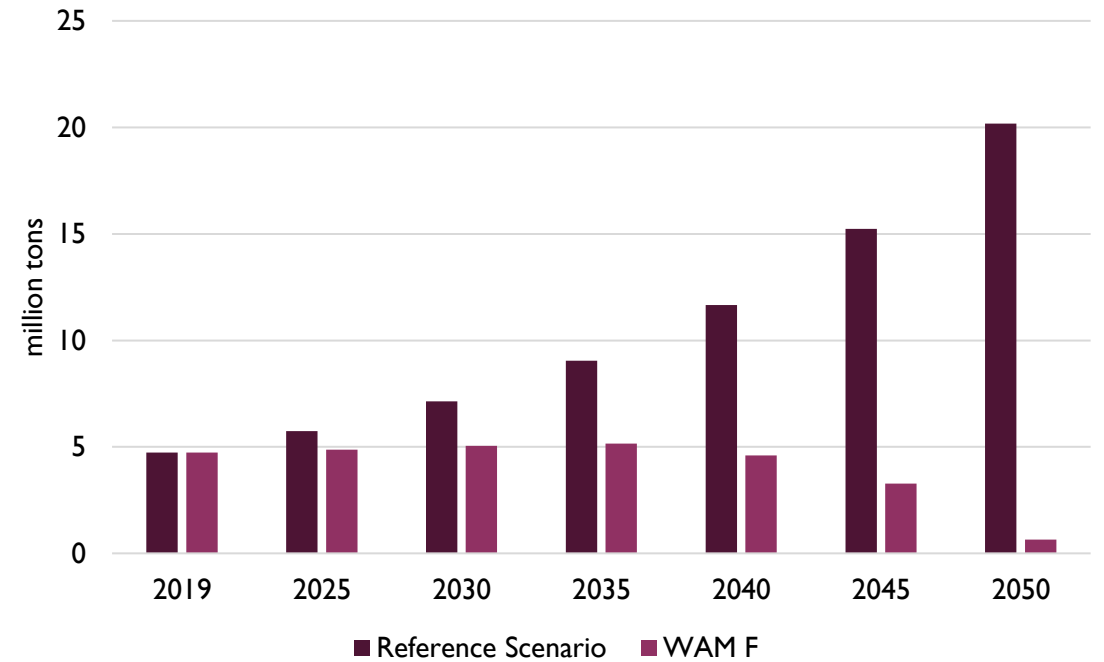
CO2 emissions
